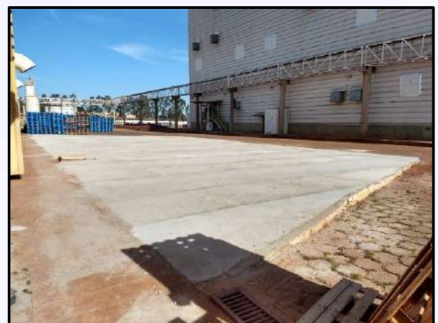
Execução de Piso de Concreto Armado
