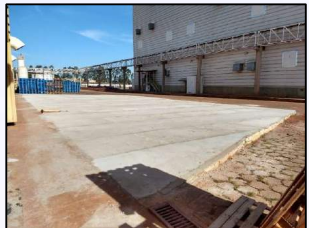
Execução de Piso de Concreto Armado em Indústria
